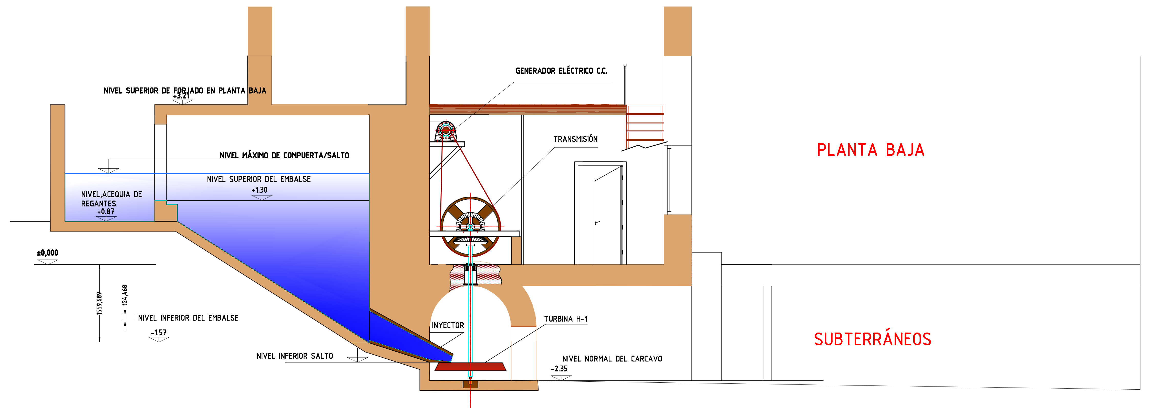
SECCION TRANSVERSAL A-A
